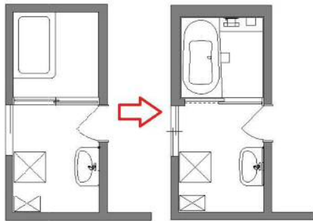
Before～After 平面図
